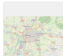
Robustesse Rennes
