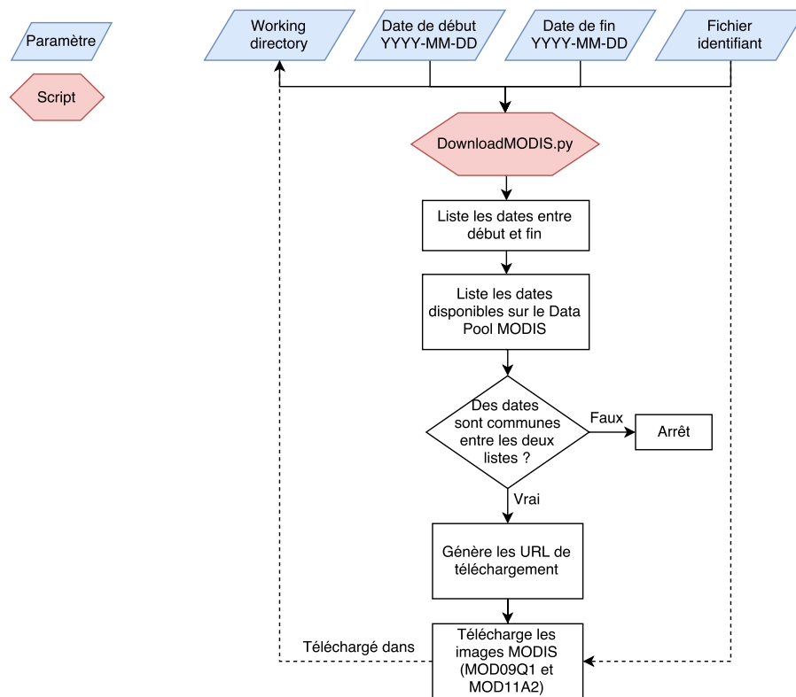
Figure 5: Organigramme du téléchargement des produits MODIS.
