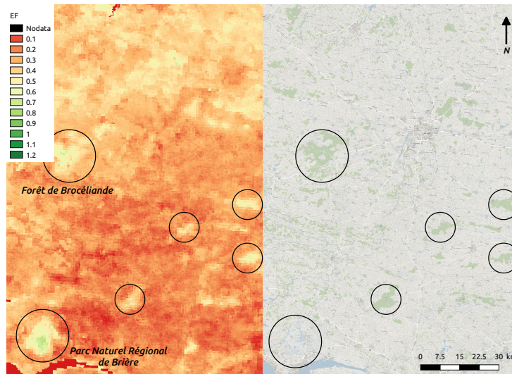
Figure 12: Evaporative Fraction au 18 Juin 2017 (à gauche) permettant de distinguer les espaces forestiers et le PNR de Brière et d'estimer le stress hydrique.
