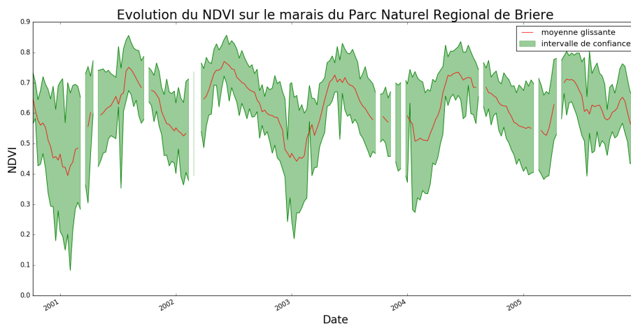
Figure 11: Représentation de l'évolution du NDVI entre début 2001 et fin 2005 sur le Parc Naturel Régional de Brière.
