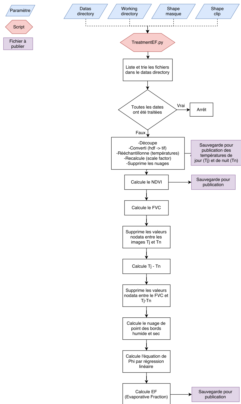
Figure 6: Organigramme de la génération des indices diffusés sur GéoBretagne.
