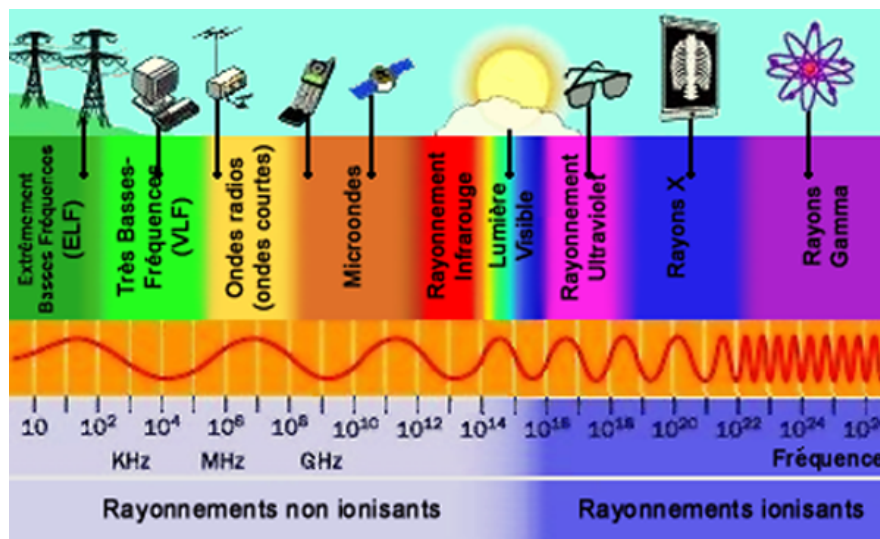
Figure 1: Représentation du spectre électromagnétique (source : astronoo.com)
