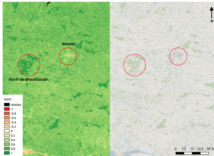
Figure 10: NDVI au 18 Juin 2017 (à gauche) permettant de distinguer les espaces forestiers, la ville de Rennes et l’embouchure de la Loire.
