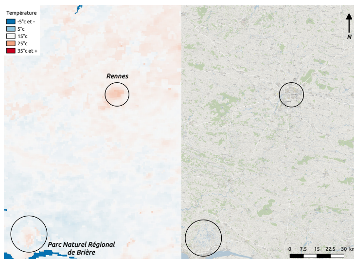
Figure 14: Température de nuit au 18 Juin 2017 (à gauche) permettant de distinguer la ville de Rennes (îlot de chaleur urbain) et le PNR de Brière.
