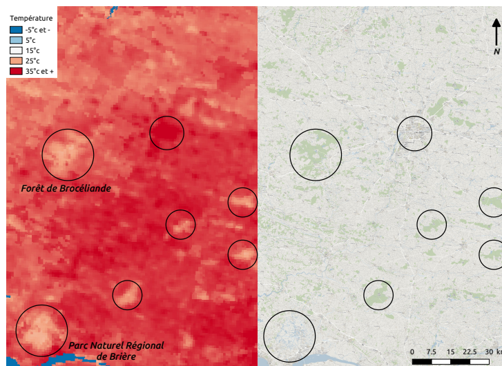
Figure 13: Température de jour au 18 Juin 2017 (à gauche) permettant de distinguer les espaces forestiers, le PNR de Brière et Rennes.
